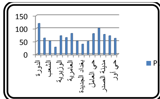
شكل ( 2 ) التمثيل البياني لتراكيز الرصاص في مناطق الدراسة لمدينة بغداد
