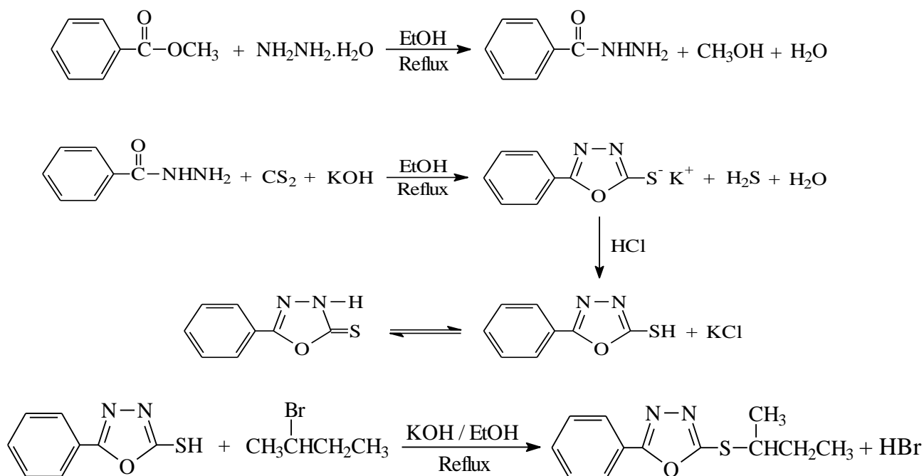
شكل (1) يبين الصيغة التركيبية للمادة الأولية والليكاند الاساس والليكاند المشتق المحضر
