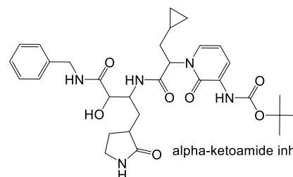
MP 576 (7)
