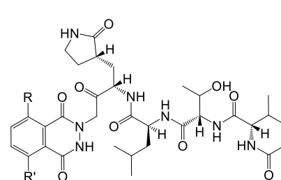
Glutamine (51-52) 51: R=R'=H 52: R= H, R'=NO 2
