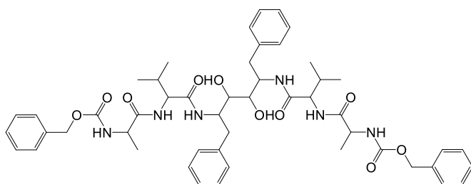
3TL (1)
