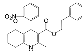
MP 576 (7)
