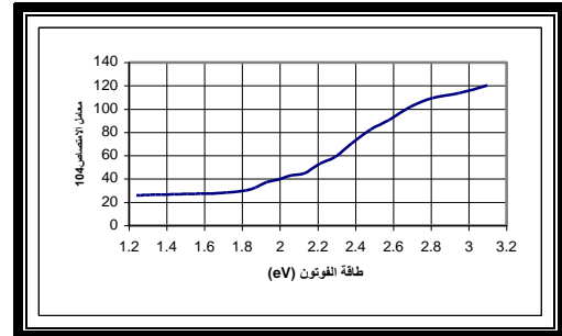
شكل(6)معامل الامتصاص كدالة لطاقة الفوتون لعشاء (CdS) بعد التشعيع بالليزر.
