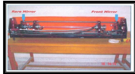
شكل رقم (1) ليزر ثاني اوكسيد الكربون
