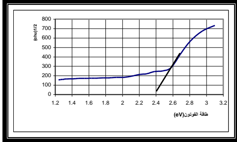
شكل (7) فجوة الطاقة المباشرة لعشاء CdS قبل التشعيع بالليزر .
