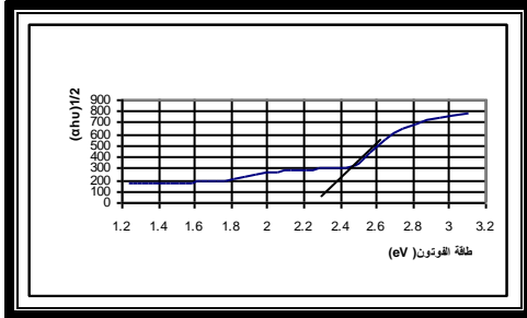
شكل (8) فجوة الطاقة المباشرة لعشاء CdS بعد التشعيع بالليزر .
